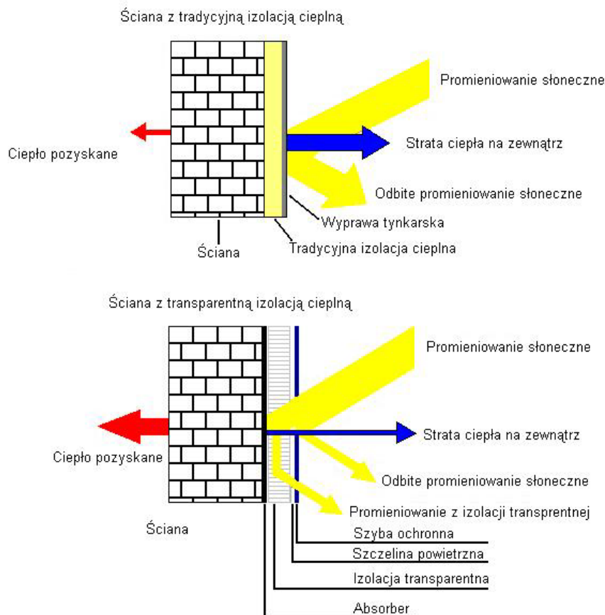
Rysunek 4 Przykład zastosowania izolacji transparentnej [23].
